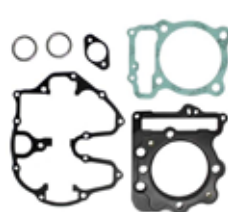
JOGO JUNTA DESCARB NX400/400i S/BORR VEDAMOTORS
